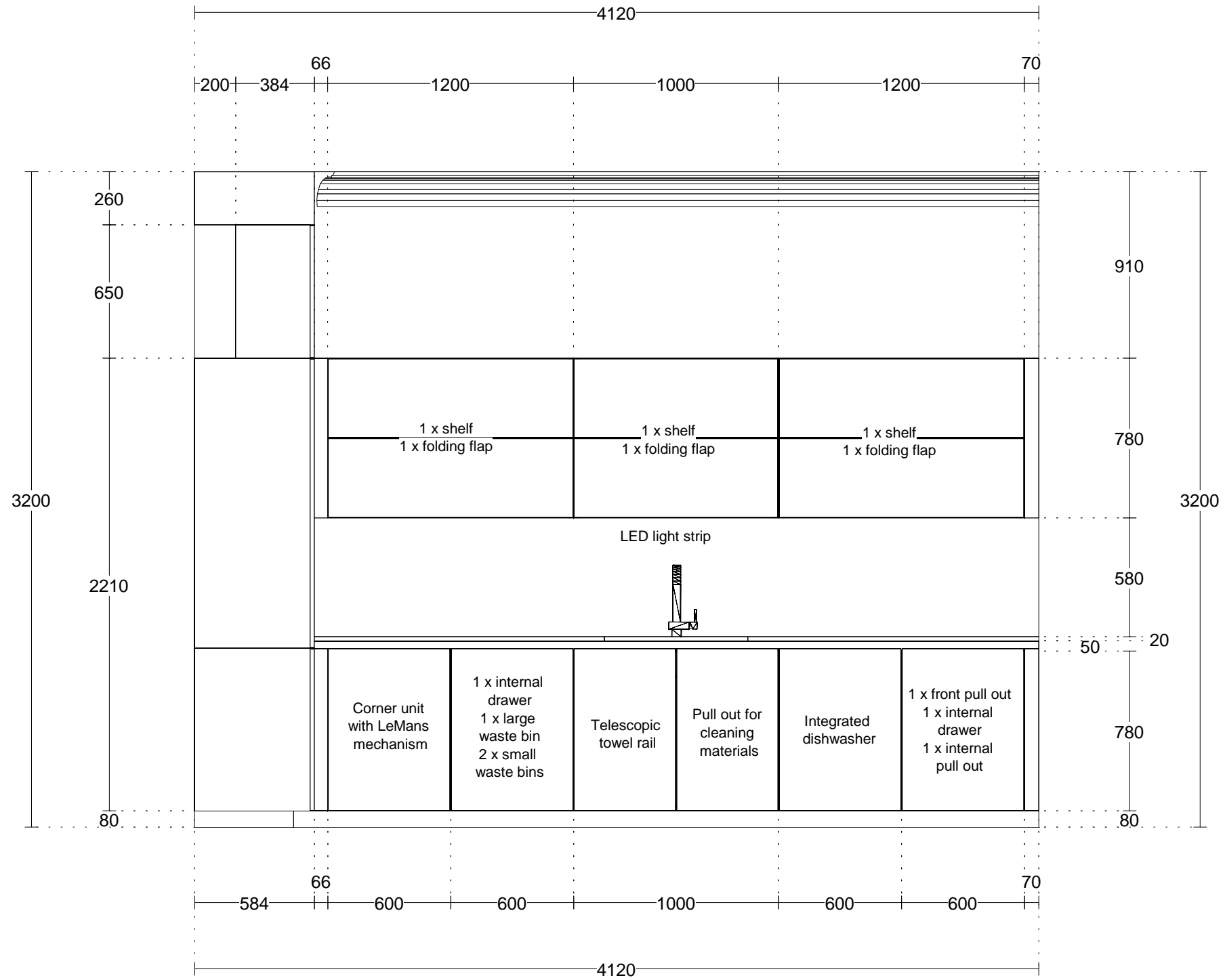
ELEVATION B
