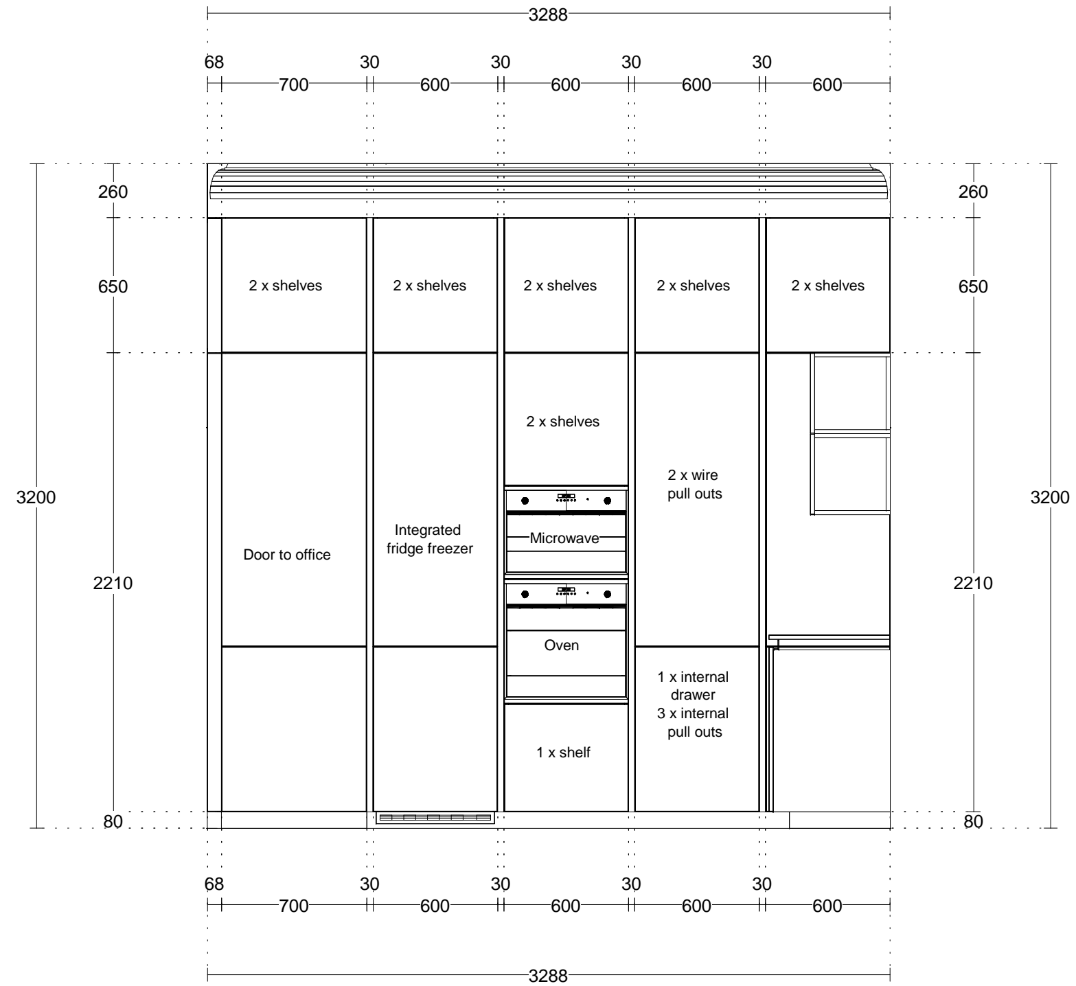
ELEVATION A
